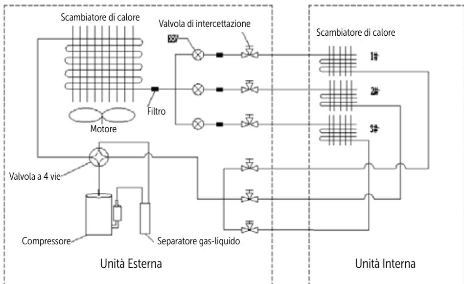
Fig.10 Schema del sistema dell'unità climatizzatore inverter MULTI-S
